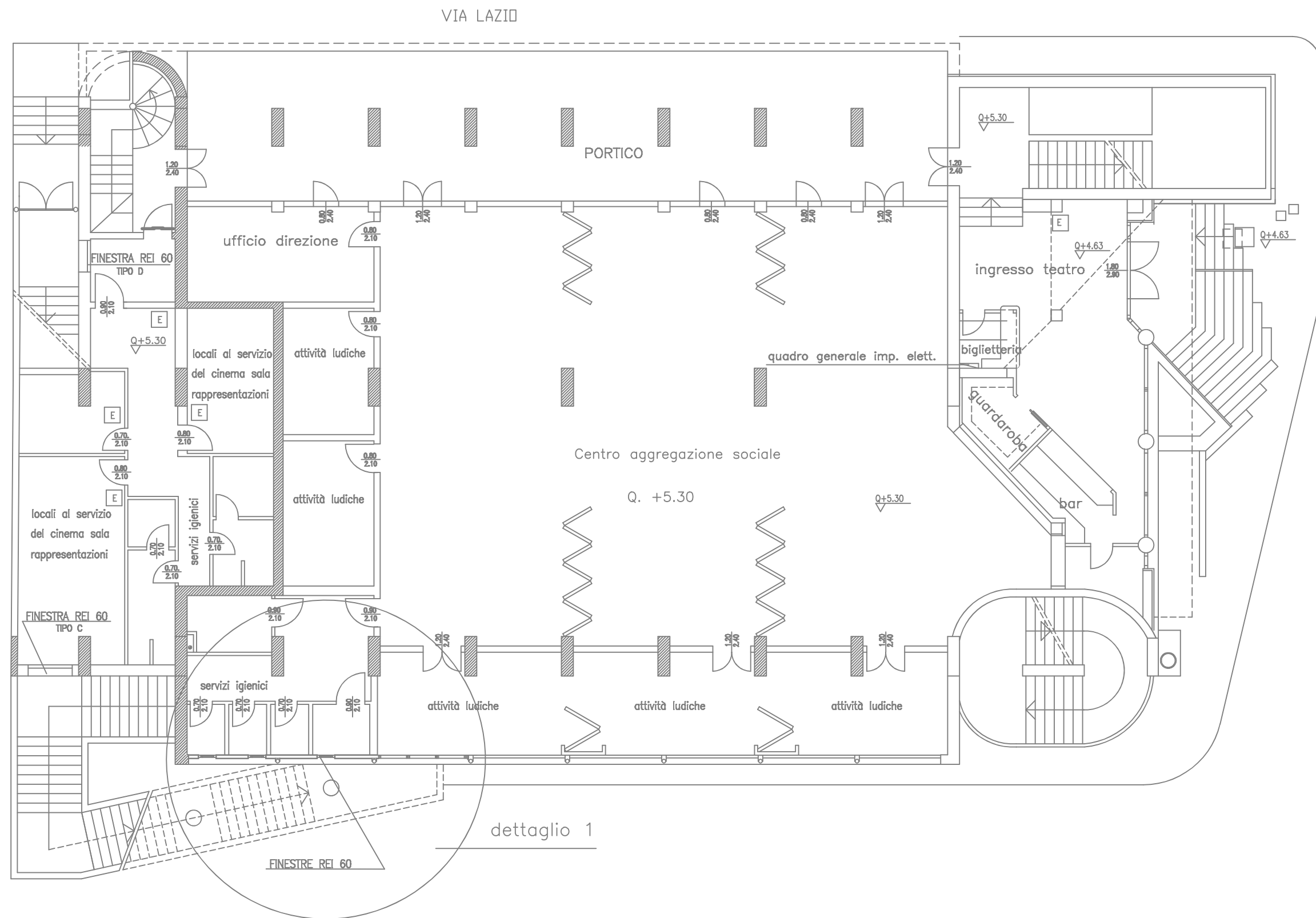
PIANTA QUOTA 5.30 – Biglietteria, Ludoteca, locali a servizio palco
